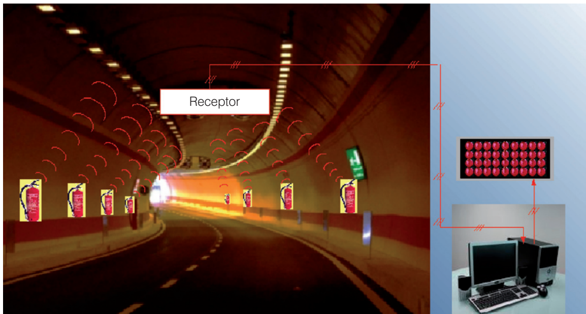
Sistema integrado de seguridad para extintores (E-SICS).
